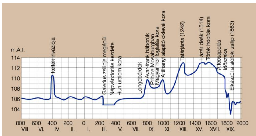
3. ábra. A Balaton vízszintingadozásai Kr.e. 800 és Kr.u. 2000 között (BENDEFY L. – V. NAGY I. 1969)
